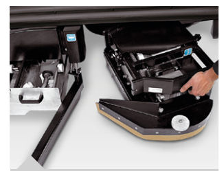
Der Grobschmutz wird von der Zylinderbürste in einen dafür vorgesehenen geräumigen Behälter gesammelt. Die Wartung der Bürsten ist dank ihrer leichten Austauschbarkeit sehr einfach
